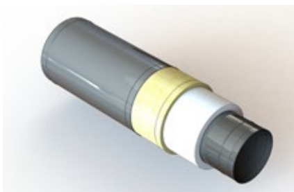
Dettaglio costruttivo del modulo DUCTFIRE M: all'interno della doppia parete metallica è interposto uno speciale accoppiato isolante ad alte prestazioni con spessore 100 mm.
